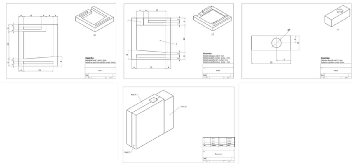
Slika 16: Delavniške risbe in sestavna risba s kosovnico (lasten vir)
