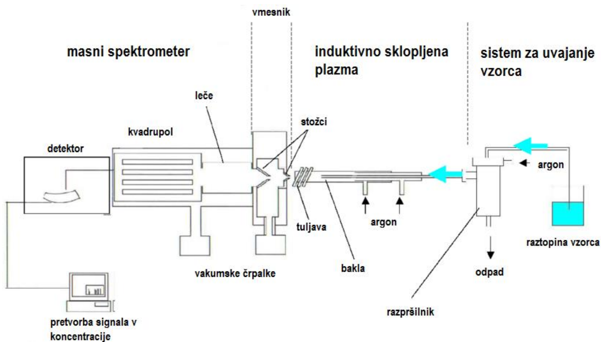
SLIKA 2: PRIKAZ OSNOVNIH KOMONENT INŠTRUMENTA ICP-MS (GILSTRAP, 2009)
