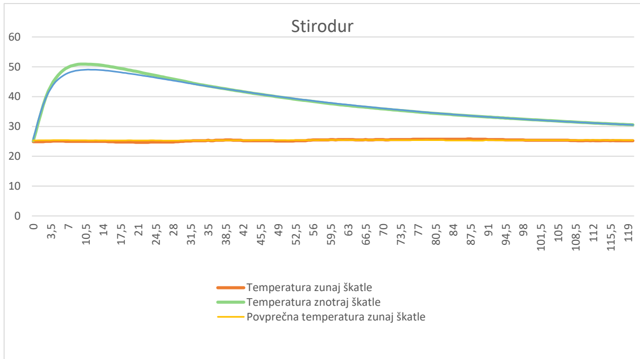
Graf 4: Rezultati za stirodur debeline 20 mm
