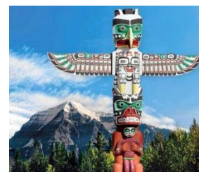
Slika 50: Totem
