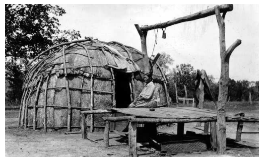
Slika 2: Vigvam
