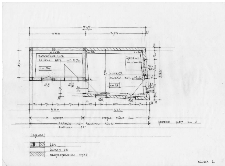
Slika 16: Načrt izgradnje bolnišnice Jesen 2
