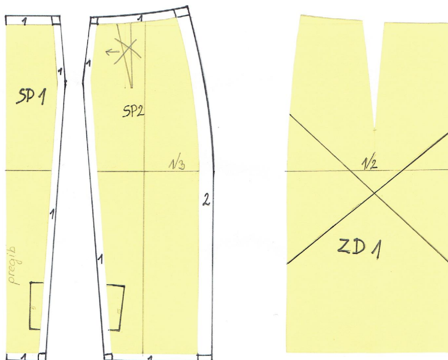
Slika 21: Modeliran kroj zgornjega krila (Vir: avtorici naloge)
