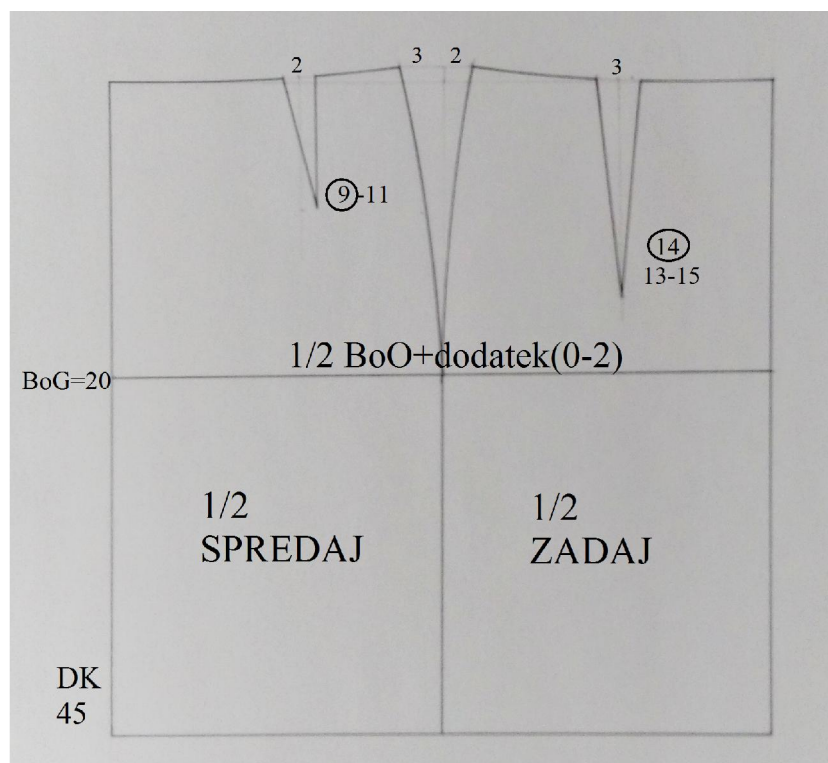
Slika 20: Osnovni kroj zgornjega krila (Vir: avtorici naloge)
