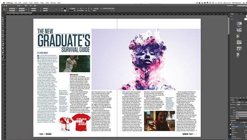
Slika 33: Adobe Indesign
