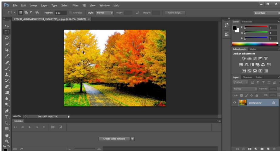
Slika 32: Adobe Photoshop
